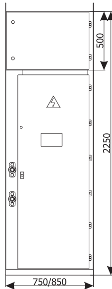
Фасад
