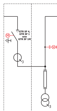
SS2L(P. *) (секционная ячейка с разъединителем или выключателем нагрузки слева)
