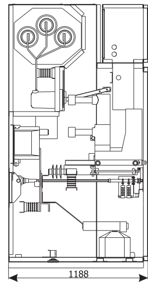
Сечение шкафа
