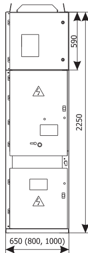
Фасад
