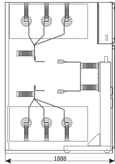
Сечение шкафа
