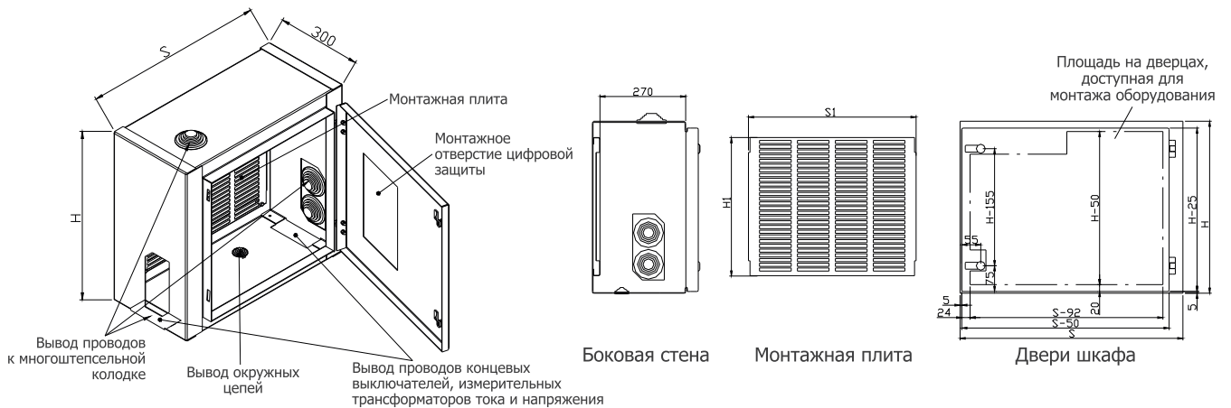
Рисунок 3а - Шкаф вспомогательных цепей в распределительном устройстве RXD
