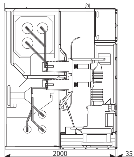
Сечение шкафа
