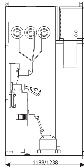
Сечение шкафа
