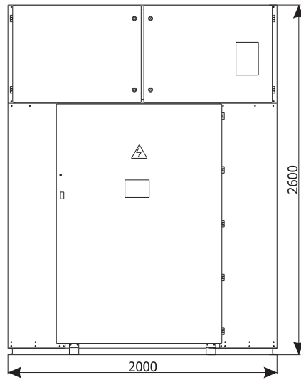
Фасад
