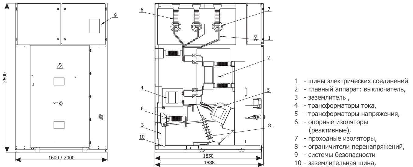
Рисунок 2 - Структурные схемы силовых цепей
