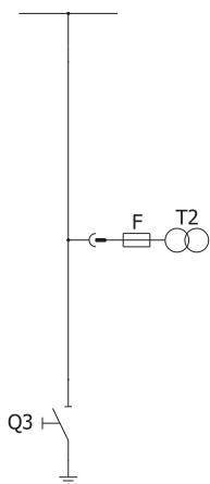
Структурная схема
