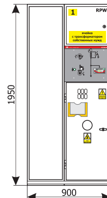
Stpwł4 (ячейка с трансформатором собственных нужд)
