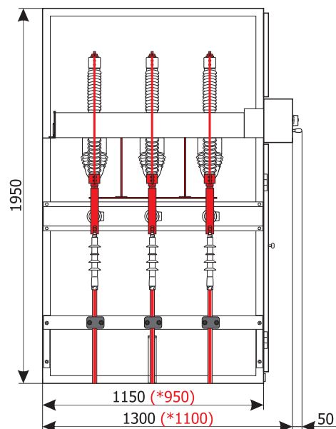
Боковой разрез
