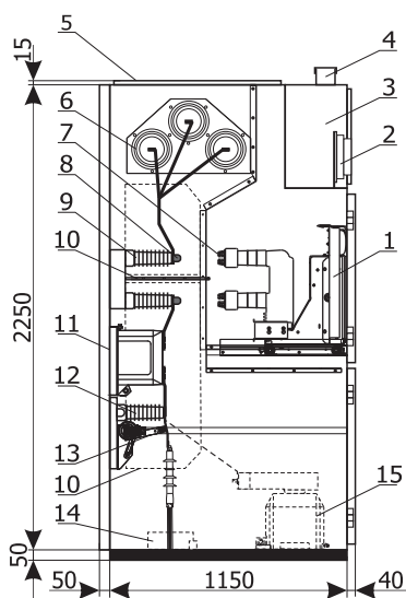
Ячейка тип RCW1
