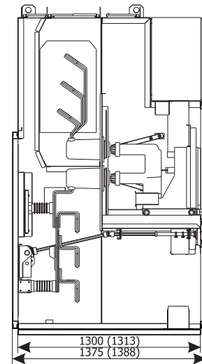
Сечение шкафа
