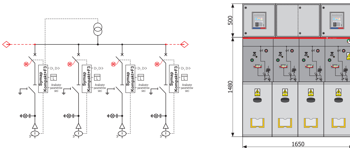
Конфигурация WWWW(4 ячейки выключателя ячейки)
