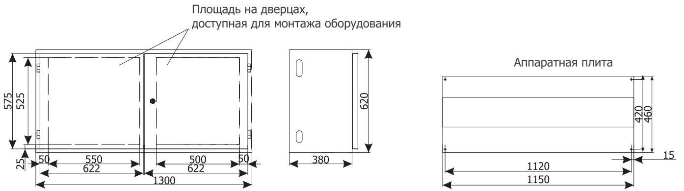
Рисунок 3б - Шкаф вспомогательных цепей ячейки RELF 3б
