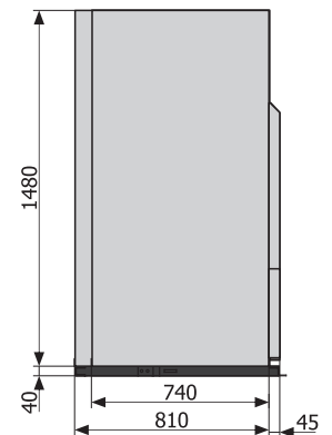
Вид сбоку
