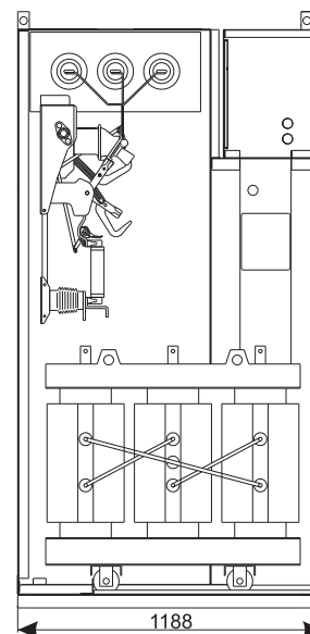
Сечение шкафа
