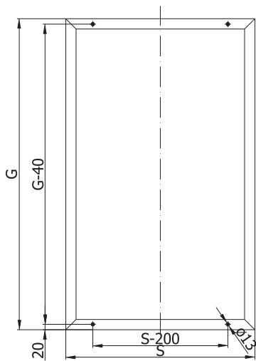
Рисунок 6а - Несущая/монтажная рама распределительного устройства RXD 12/17,5/24
