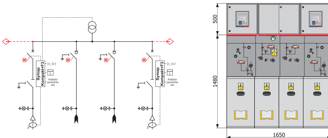
Конфигурация WWWW(4 ячейки выключателя ячейки)
