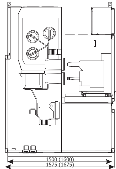
Сечение шкафа
