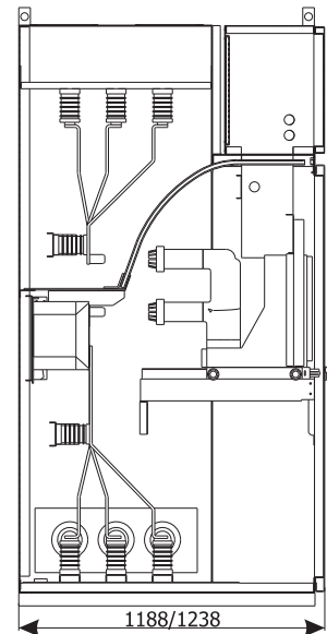
Сечение шкафа
