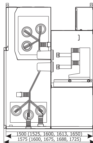
Сечение шкафа
