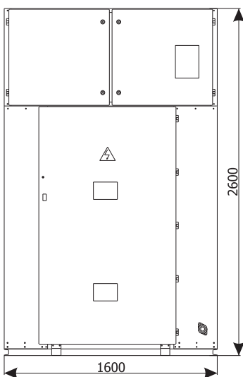
Фасад
