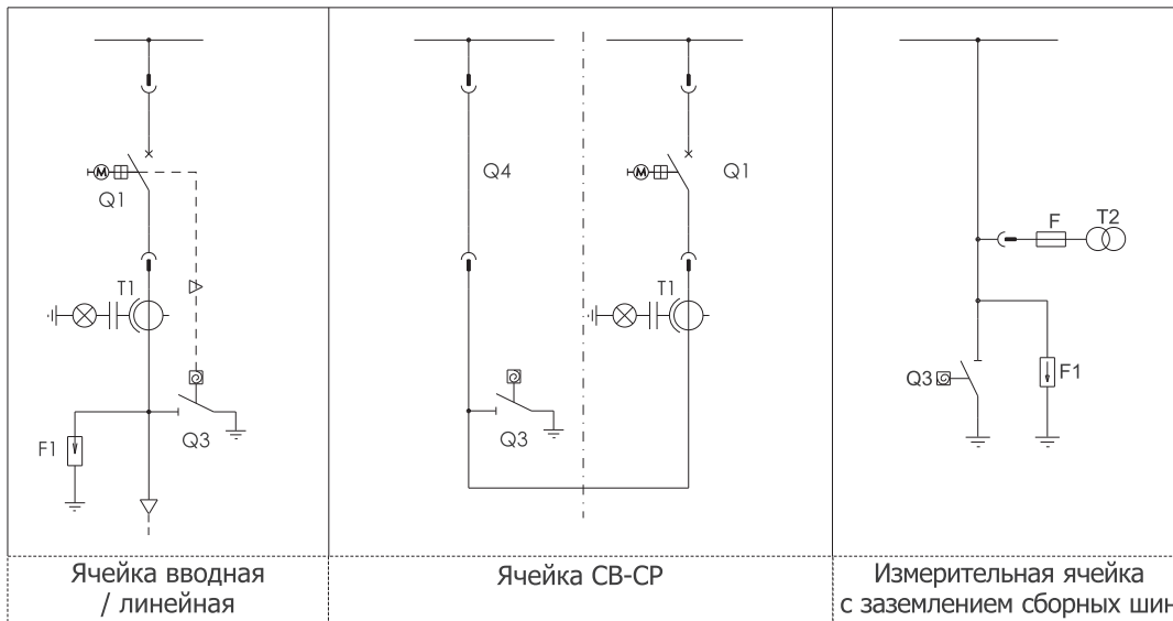
Рисунок 2б - Структурные схемы силовых цепей RELF 3б
