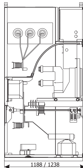
Сечение шкафа
