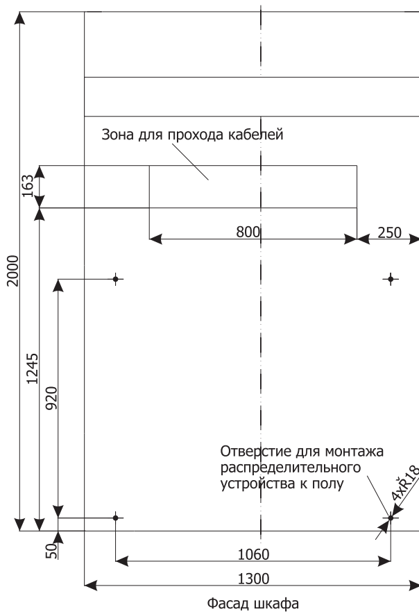
Рисунок 6в - Примерные размеры площади оснований шкафов и отверстий пола для ячеек RELF ex
