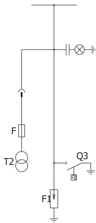
Структурная схема
