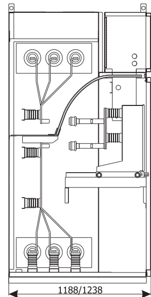
Сечение шкафа
