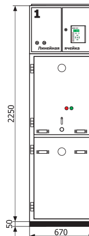
Вид спереди
