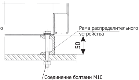
Крепление к стальной конструкции
