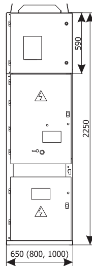
Фасад
