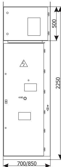
Фасад
