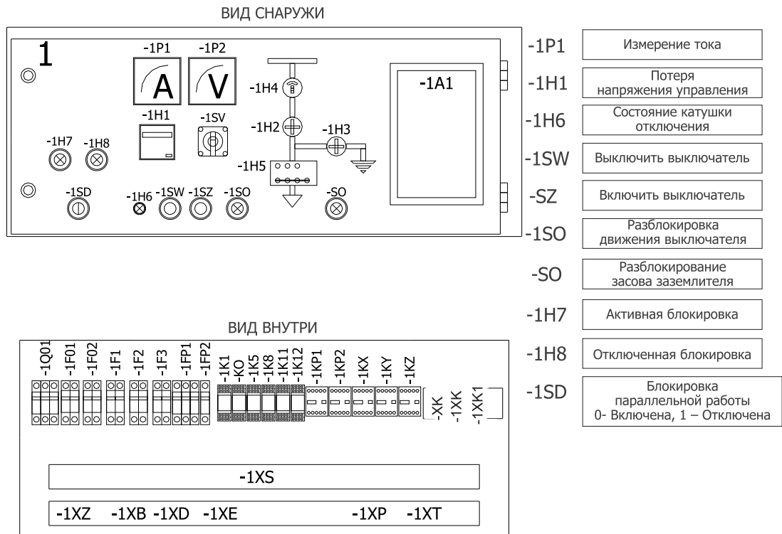
Рисунок 4б - Пример размещения аппаратуры в отсеке вспомогательных цепей ячеек RELF ex
