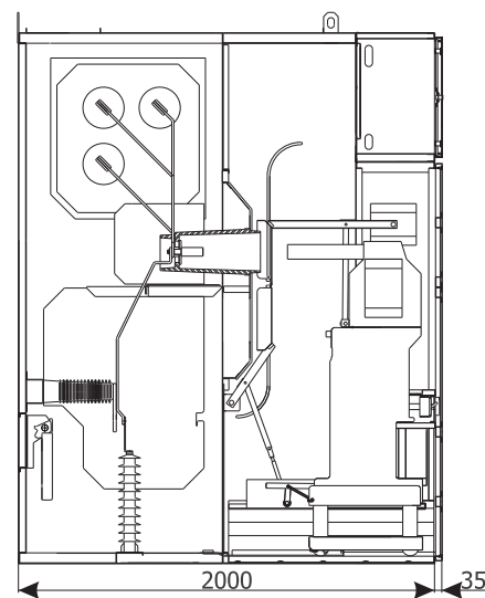
Сечение шкафа
