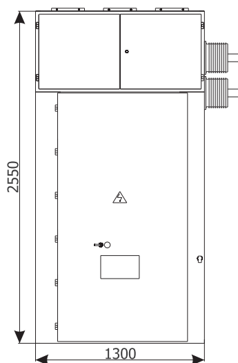
Фасад
