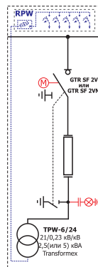
Stpwł4 (ячейка с трансформатором собственных нужд)
