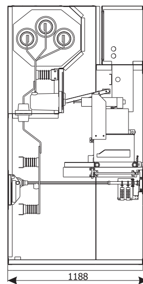
Сечение шкафа
