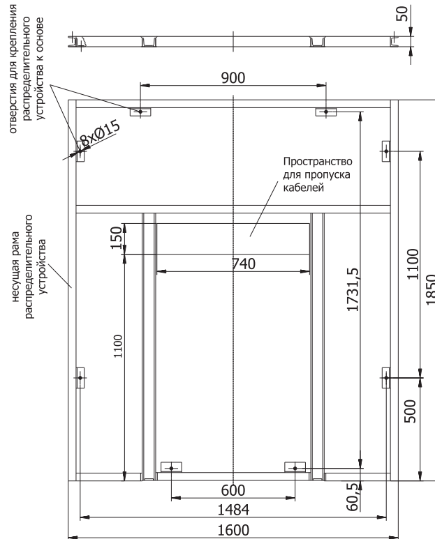
Рисунок 6б - Несущая/монтажная рама распределительного устройства RXD 36
