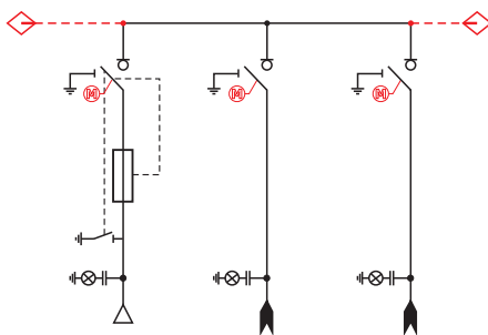
Конфигурация TLL(трансформаторная и 2 линейные ячейки)
