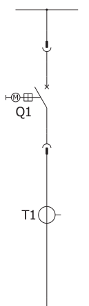
Структурная схема
