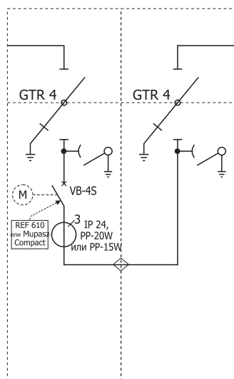
Электрическая схема
