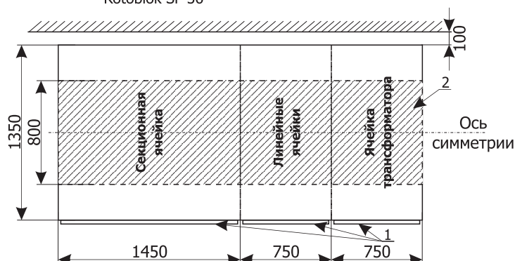
Рис 2 Пример выполнения кабельного канала под распределительным устройством Rotoblok SF 36
