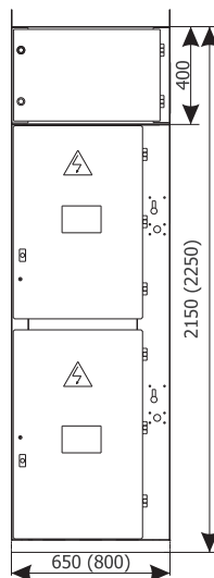
Фасад
