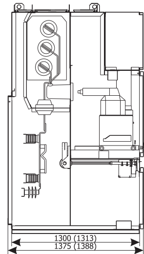
Сечение шкафа
