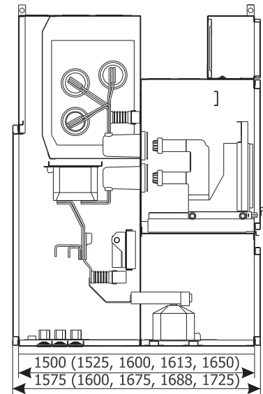
Сечение шкафа
