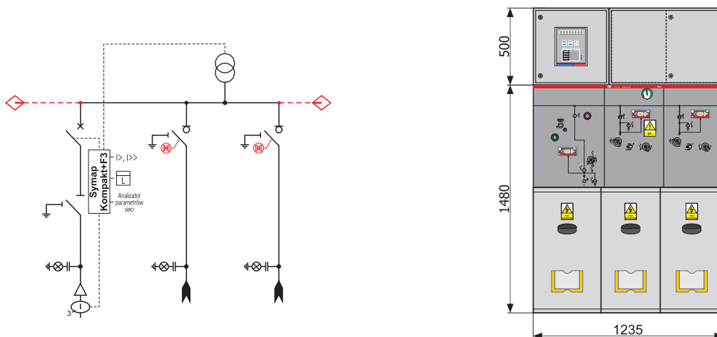
Конфигурация WLLW(2 ячейки выключателя и 2 линейные ячейки)
