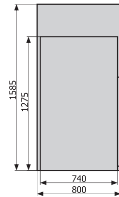
Вид сбоку
