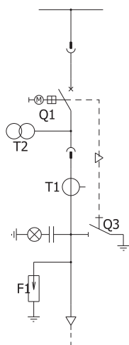
Структурная схема
