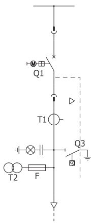
Структурная схема
