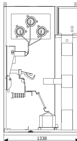
Сечение шкафа
