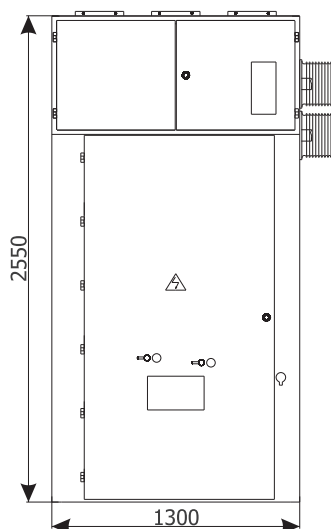
Фасад
