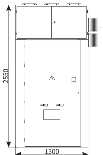
Фасад
