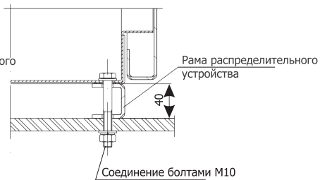
Крепление к стальной конструкции
