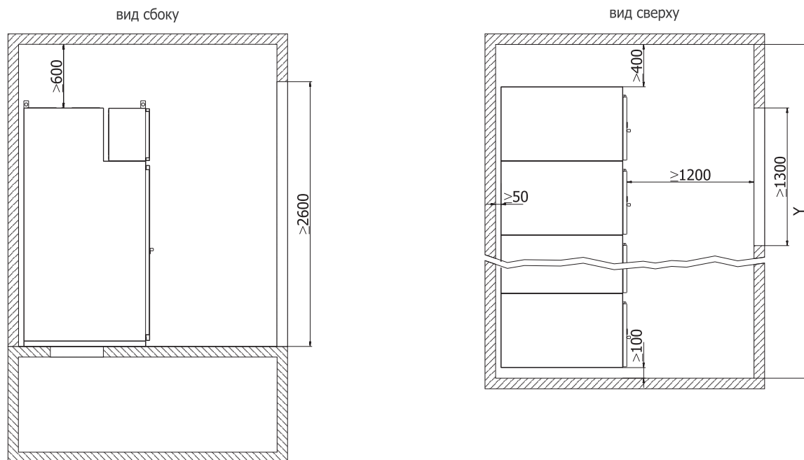
Рисунок 5б - Установка распределительного устройства RXD 36
