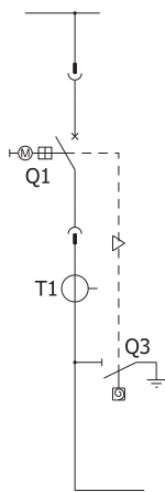
Структурная схема
